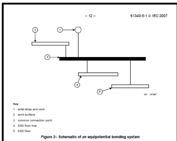
Figura 2 – schema di “equipotential bonding” – ref. IEC 61340-5-1
